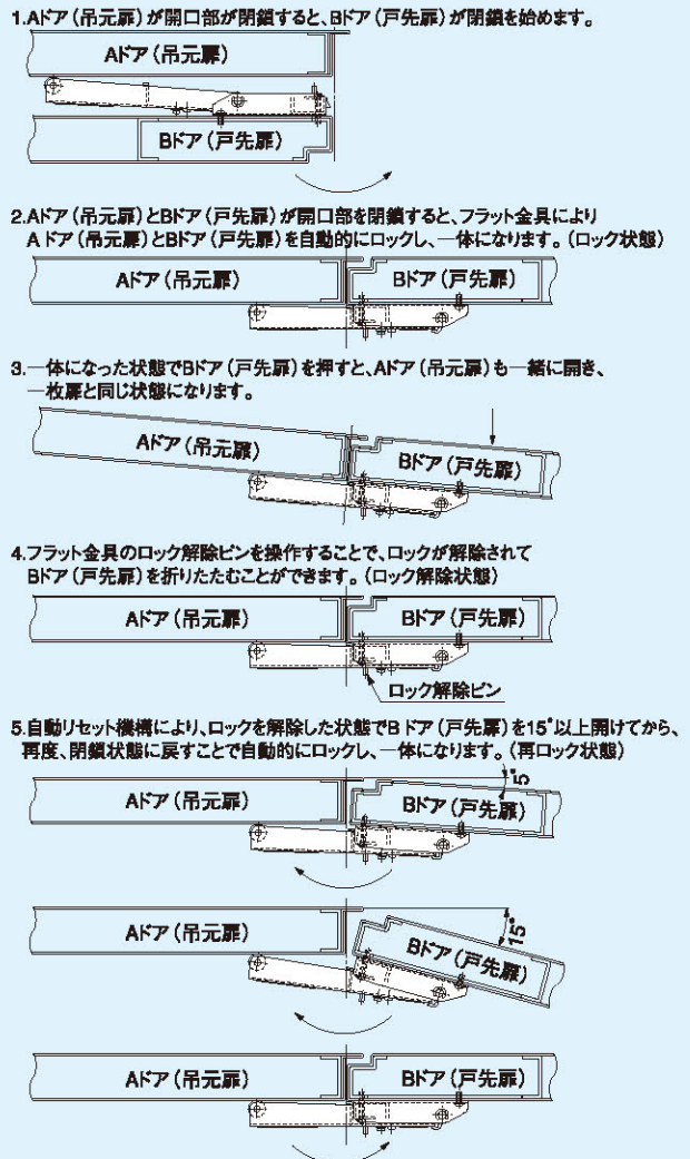
作動説明図
