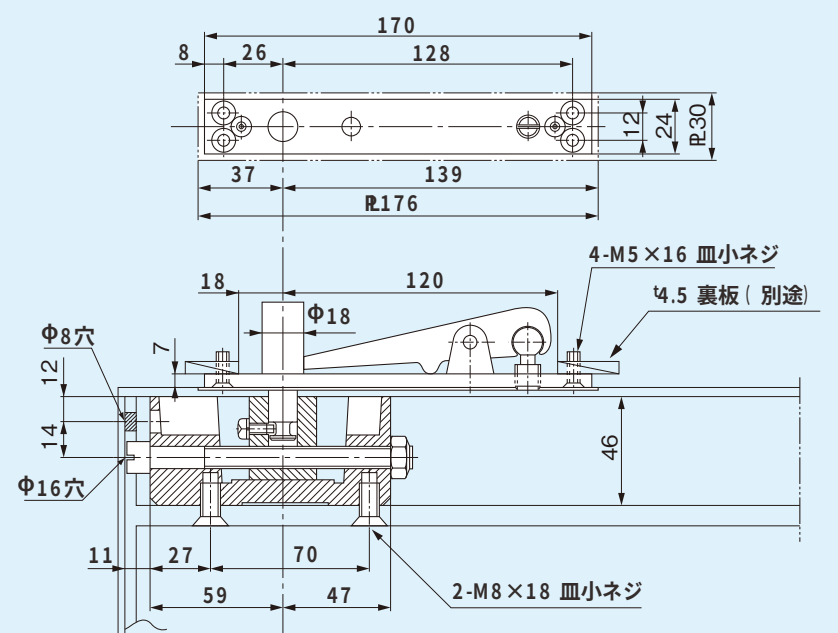
1 トップピボット (上枠側)
