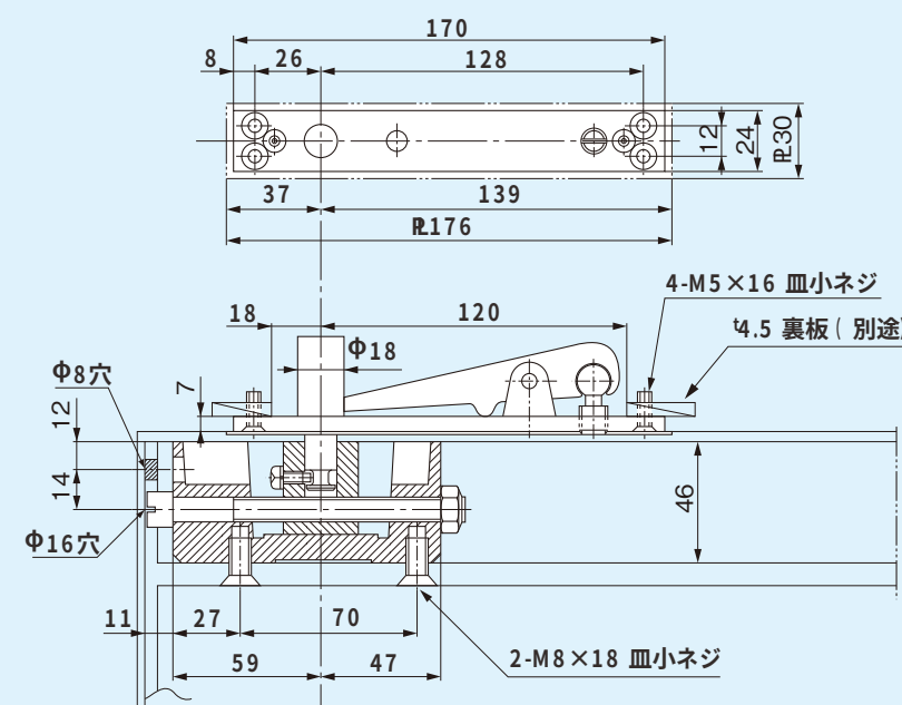
1 トップピボット (上枠側)
