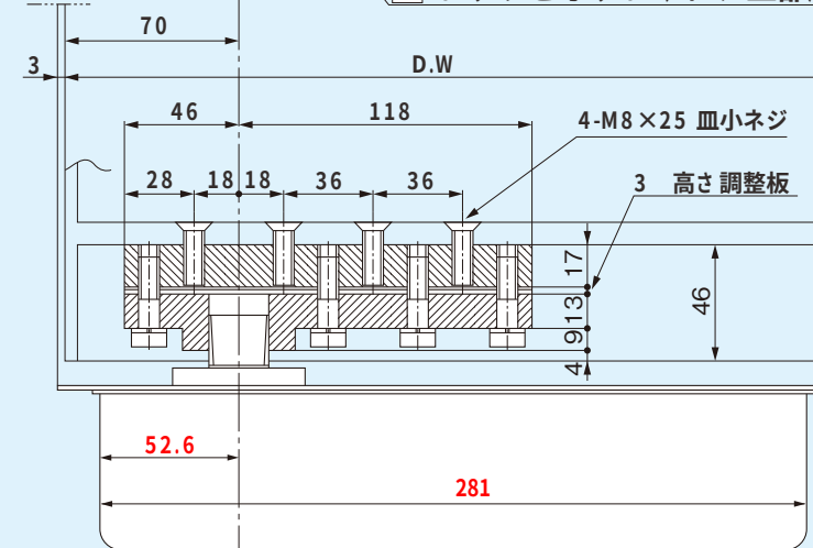
2 トップピボット (ドア上部)
