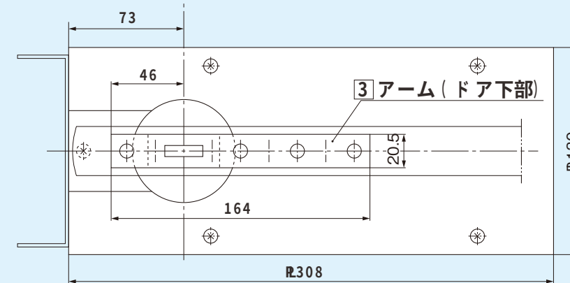
4 フロアヒンジ部品ナシ本体 (床側)
