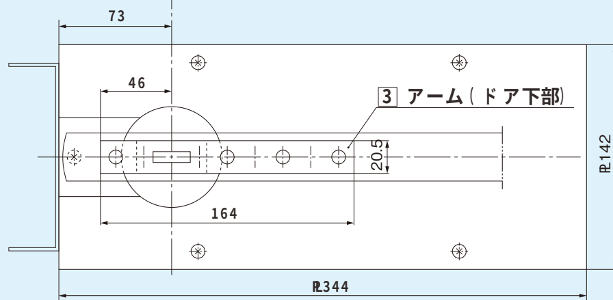
4 フロアヒンジ部品ナシ本体 (床側)
