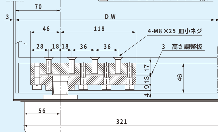
2 トップピボット (ドア上部)
